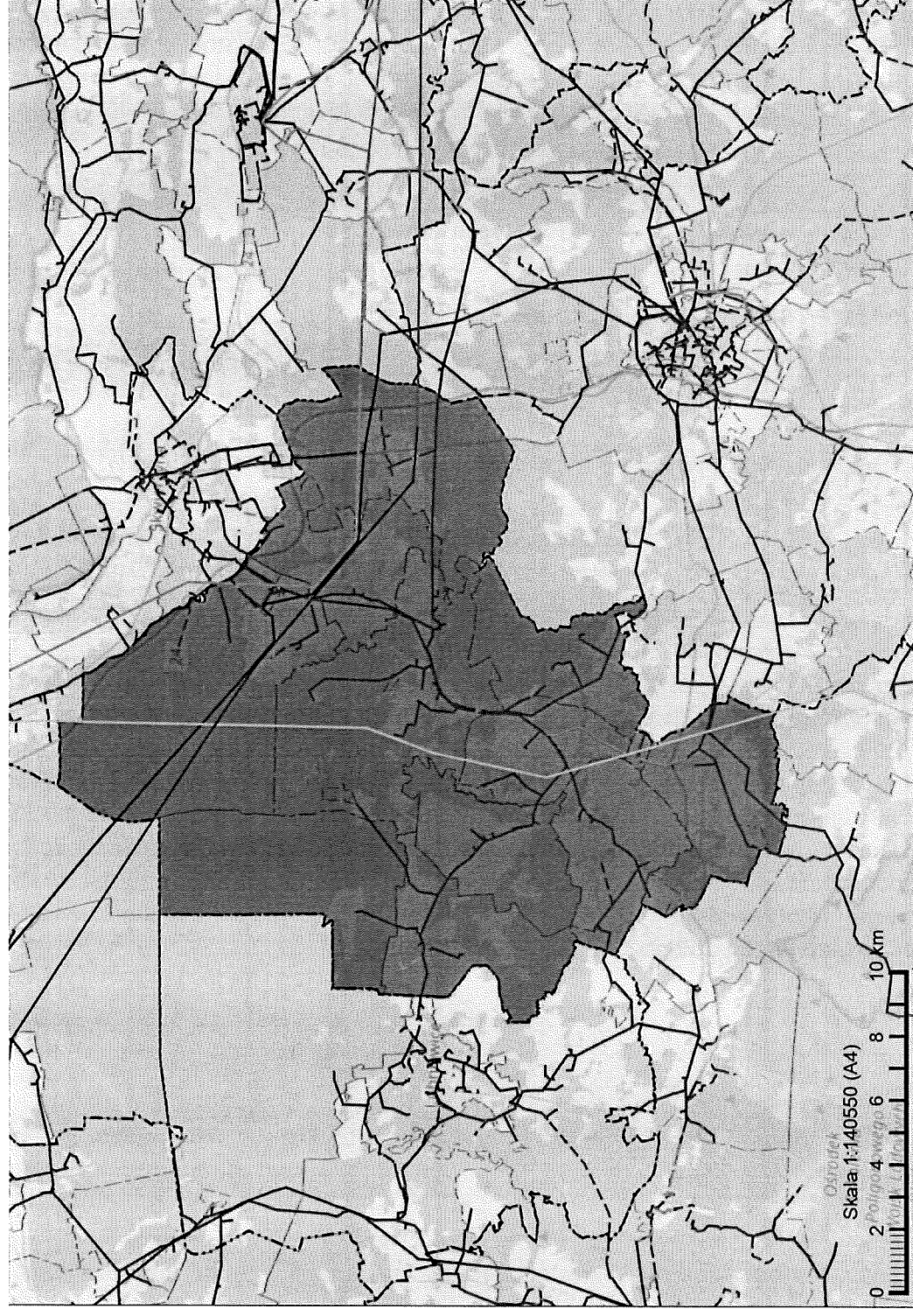
Rysunek 9. Mapa sieci 15 kV na terenie Gminy Bledzew. Źródło: ENEA Operator Sp. z o.o. Oddział Dystrybucji Gorzów Wielkopolski
