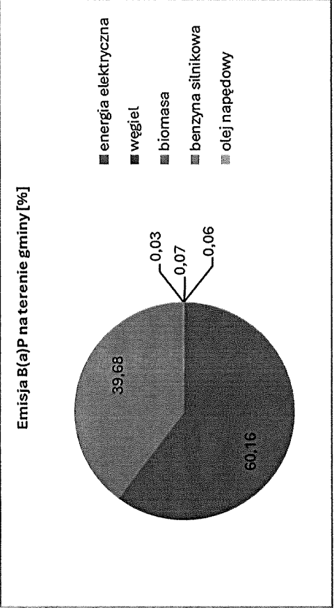
Rysunek 51. Sumaryczna emisja B(a)P wg rodzajów paliw w roku 2020 (%)
