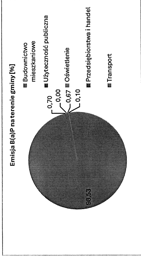
Rysunek 53. Sumaryczna emisja B(a)P wg sektorów w roku 2016 (%).
