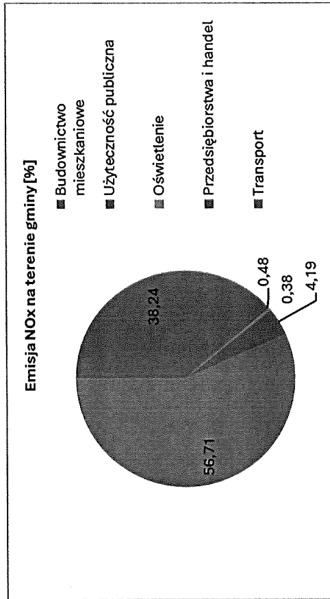
Rysunek 37. Sumaryczna emisja NOx wg sektorów w roku 2024 (%).
