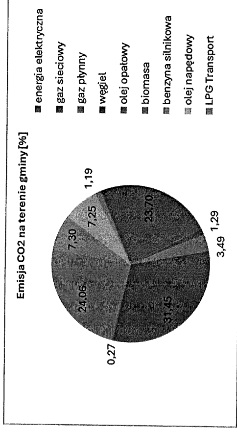
Rysunek 24. Sumaryczna emisja CO 2 wg rodzajów paliw w roku 2020 (%).
