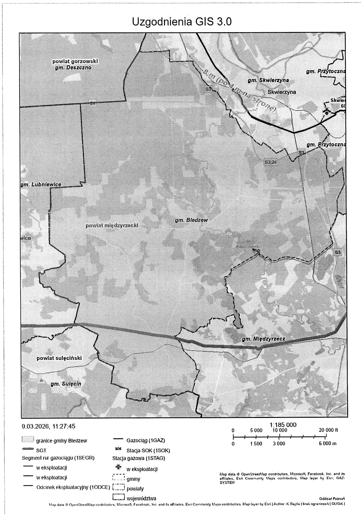
Rysunek 12. Sieć gazowa wysokiego ciśnienia na terenie Gminy Bledzew. Źródło: GAZ-SYSTEM S.A.
