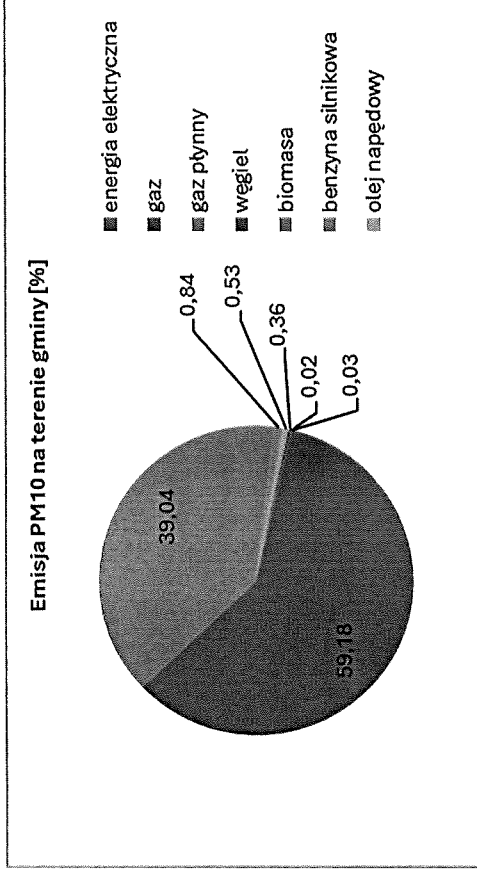
Rysunek 39. Sumaryczna emisja PM10 wg rodzajów paliw w roku 2020 (%)
