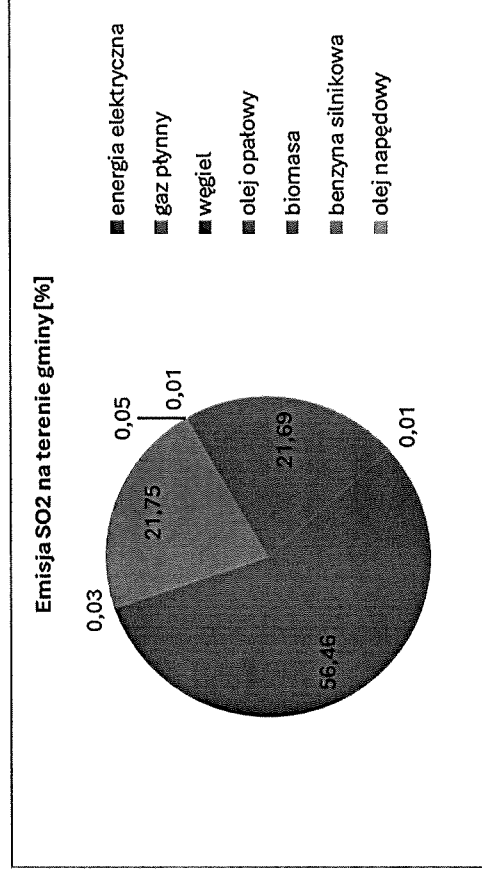
Rysunek 28. Sumaryczna emisja SO 2 wg rodzajów paliw w roku 2024 (%).
