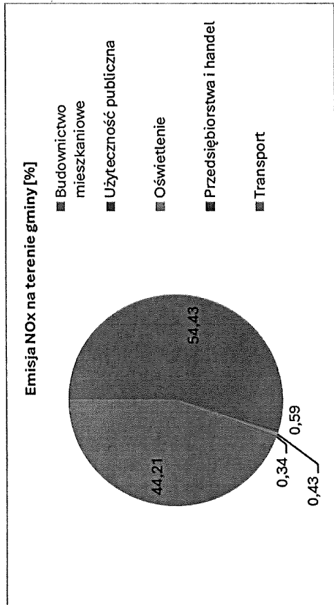
Rysunek 35. Sumaryczna emisja NOx wg sektorów w roku 2016 (%).
