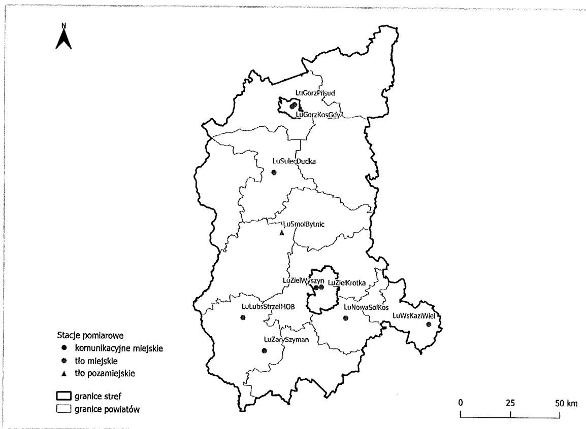
Rysunek 14. Stacje pomiarowe na terenie województwa lubuskim w roku 2024 r.
