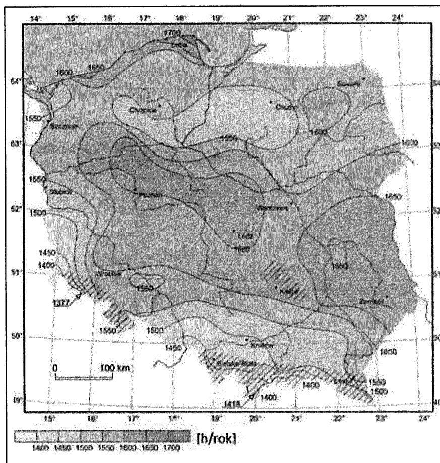
Rysunek 17. Średni czas nasłonecznienia w ciągu roku na terenie Polski [h/rok]. źródło: Urząd Regulacji Energetyki
