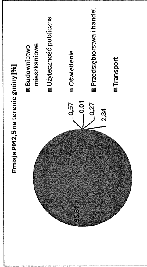
Rysunek 49. Sumaryczna emisja PM 2,5 wg sektorów w roku 2024 (%).
