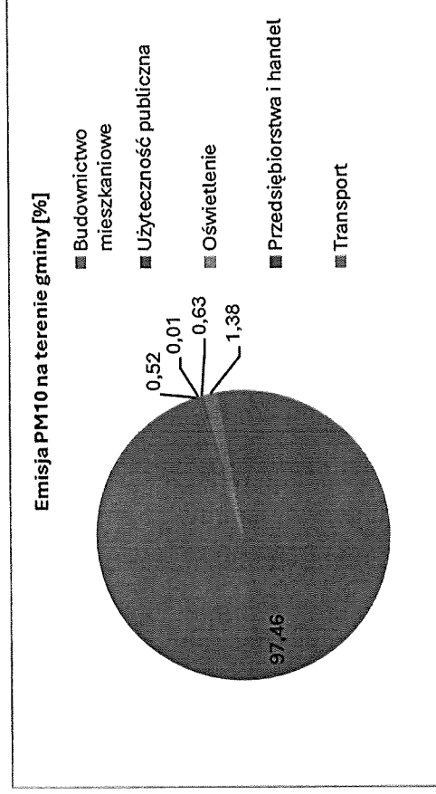
Rysunek 42. Sumaryczna emisja PM10 wg sektorów w roku 2020 (%).
