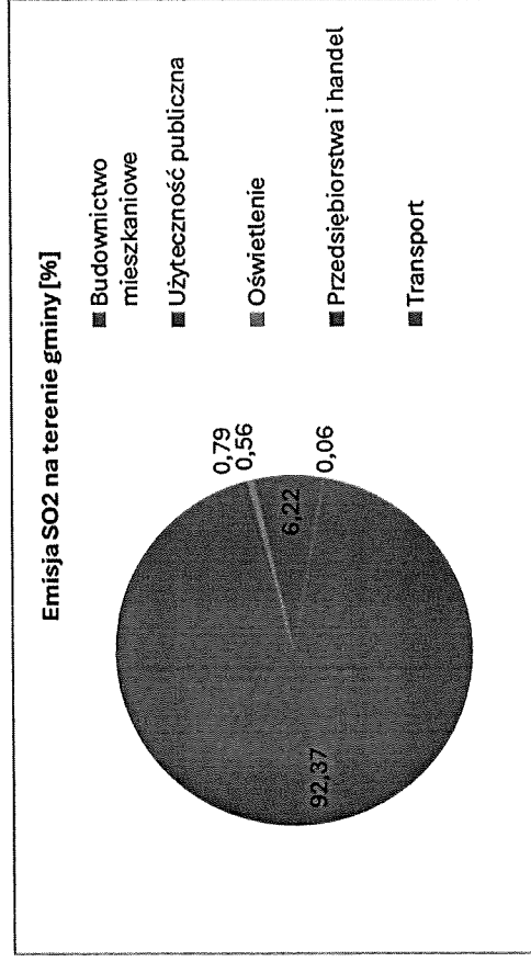
Rysunek 31. Sumaryczna emisja SO 2 wg sektorów w roku 2024 (%).
