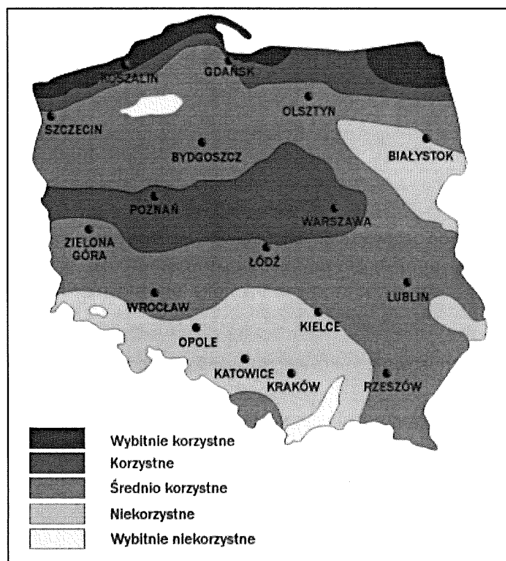
Rysunek 16. Strefy energetyczne warunków wiatrowych. źródło: IMGW
